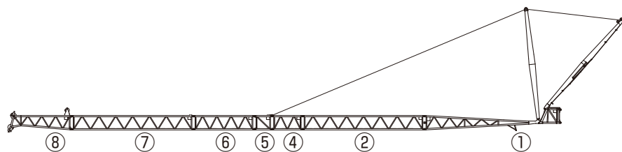
2.5m+52mジブ(ライト)
